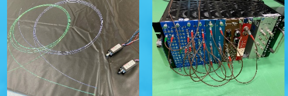
放射線検出用光ファイバ、光検出器、信号処理回路
