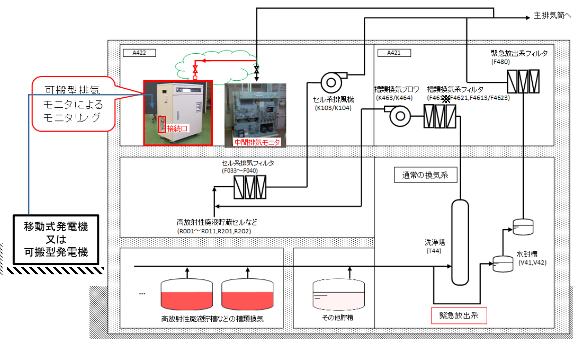
可搬型モニタリング設備への接続口設置イメージ図
