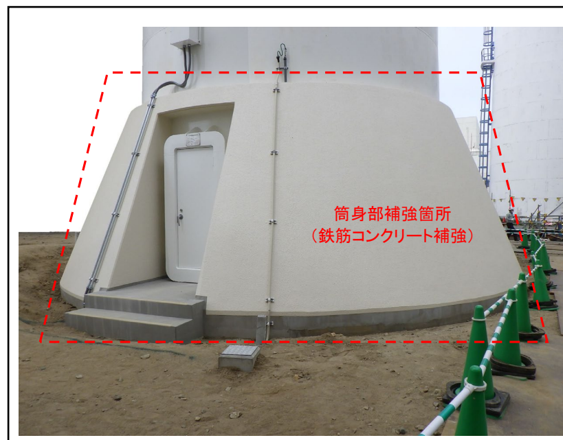
図1 第二付属排気筒の耐震補強
