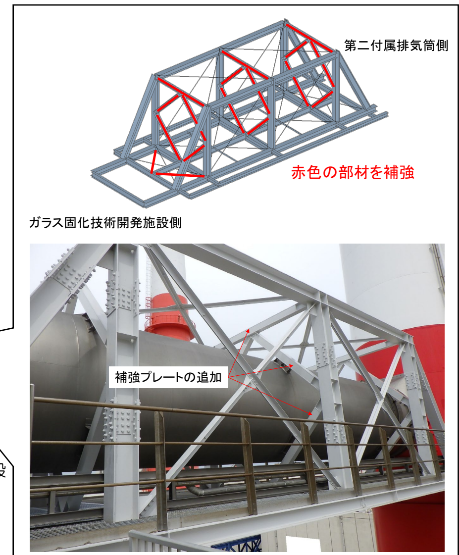
図2 排気ダクト接続架台の耐震補強
