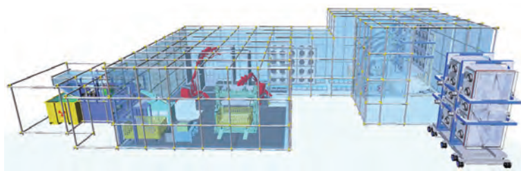
▲アドバンスドスマートデコミッションングシステムによるグローブボックスの解体イメージ
