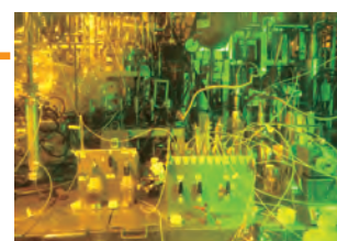
▲抽出クロマトグラフィーを用いたMA分離試験
