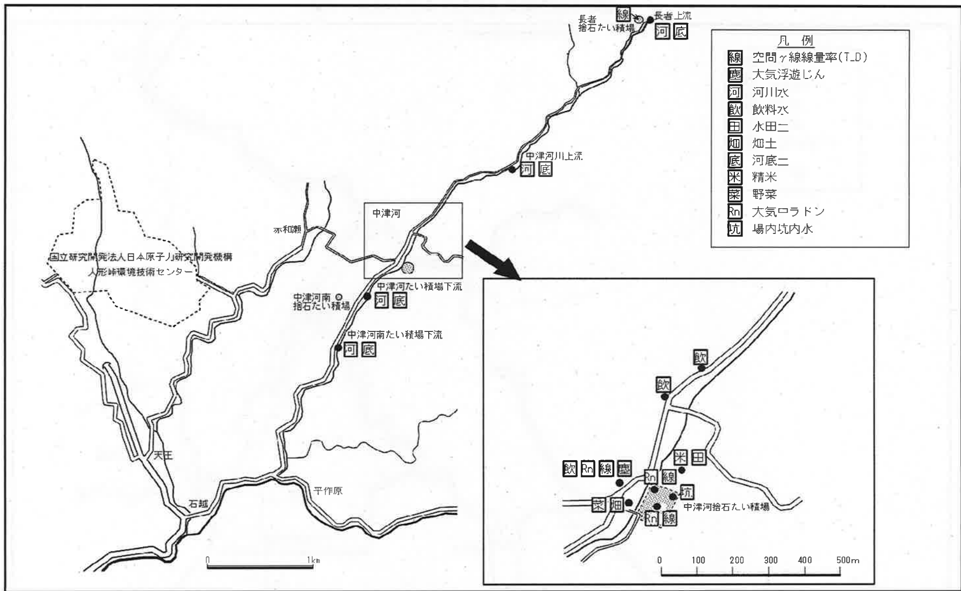
図2. 中津河捨石たい積場周辺等に係る環境放射線等監視測定地点図
