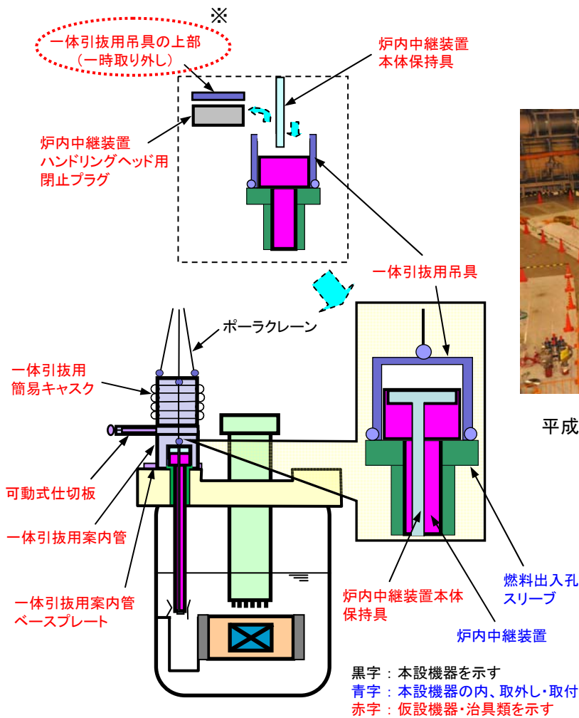
【一体引拔用吊具の上部取付け作業】
