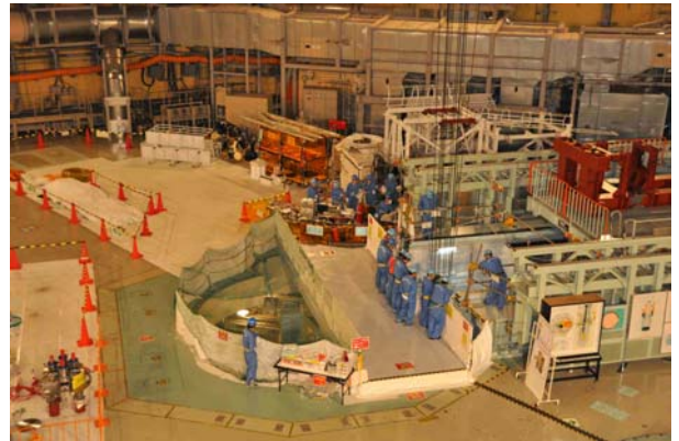
平成23年 6月17日 14時30分頃の作業風景
