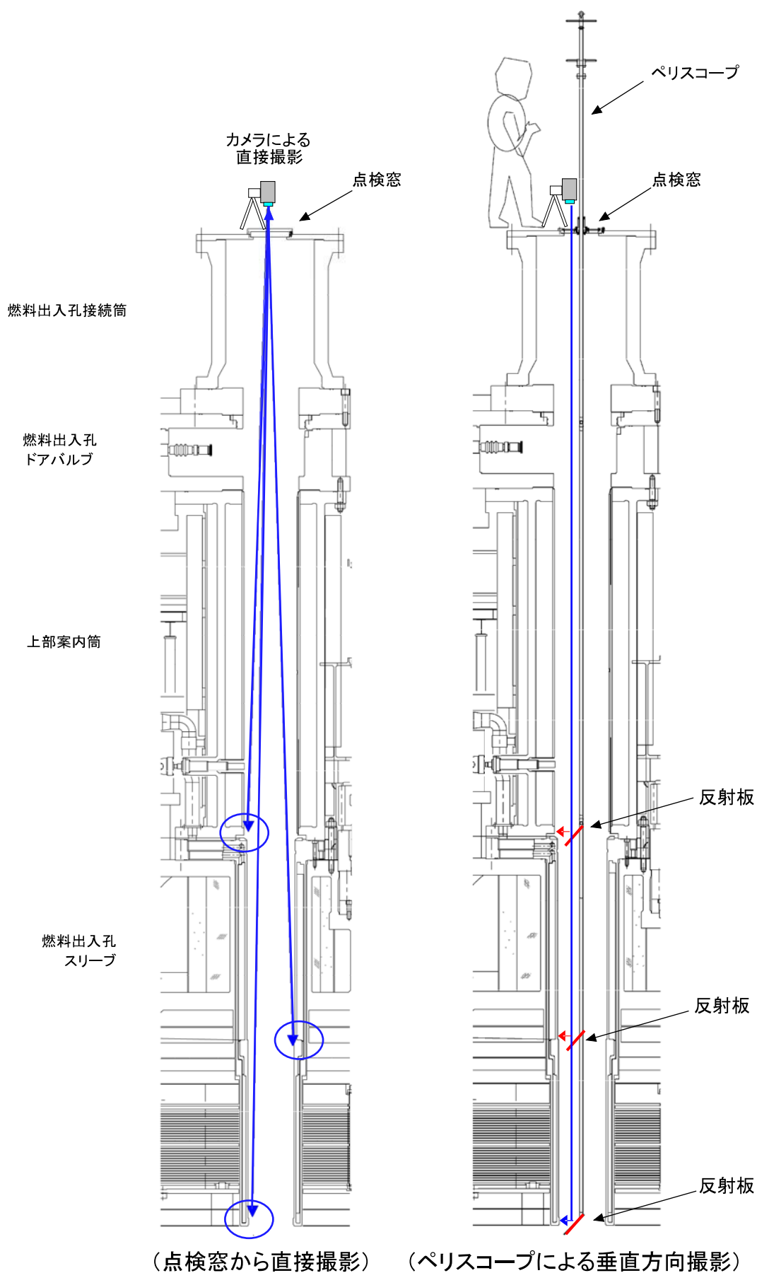
図14-5 IVTM本体引き抜き後のIVTM本体着座面及び燃料出入孔スリーブ観察方法の概要
