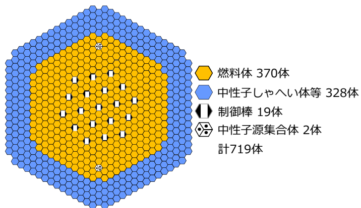
第1段階開始時炉心配置図
