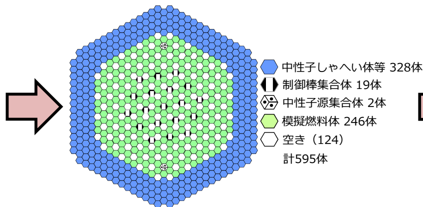
第2段階開始時炉心配置図 (現在の状態)
