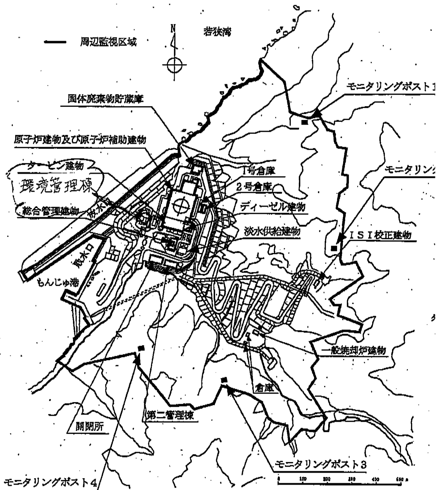
高速増殖原型炉もんじゅ 全体地図
