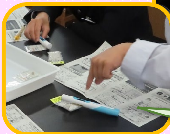
霧箱での放射線飛跡の観察
