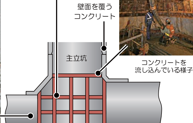
【深度500mの主立坑のイメージ図】
