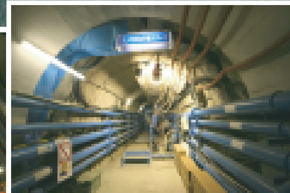
主立坑と換気立坑をつなぐ深さ100m 地点の水平の坑道（予備ステージ）
