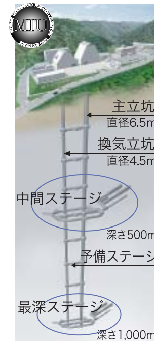
瑞浪超深地層研究所イメージ (施設の形状、配置などは変更の可能性があります)
