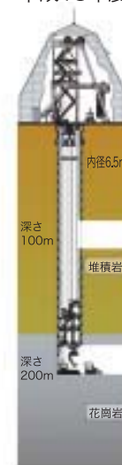
主立坑掘削のイメージ
