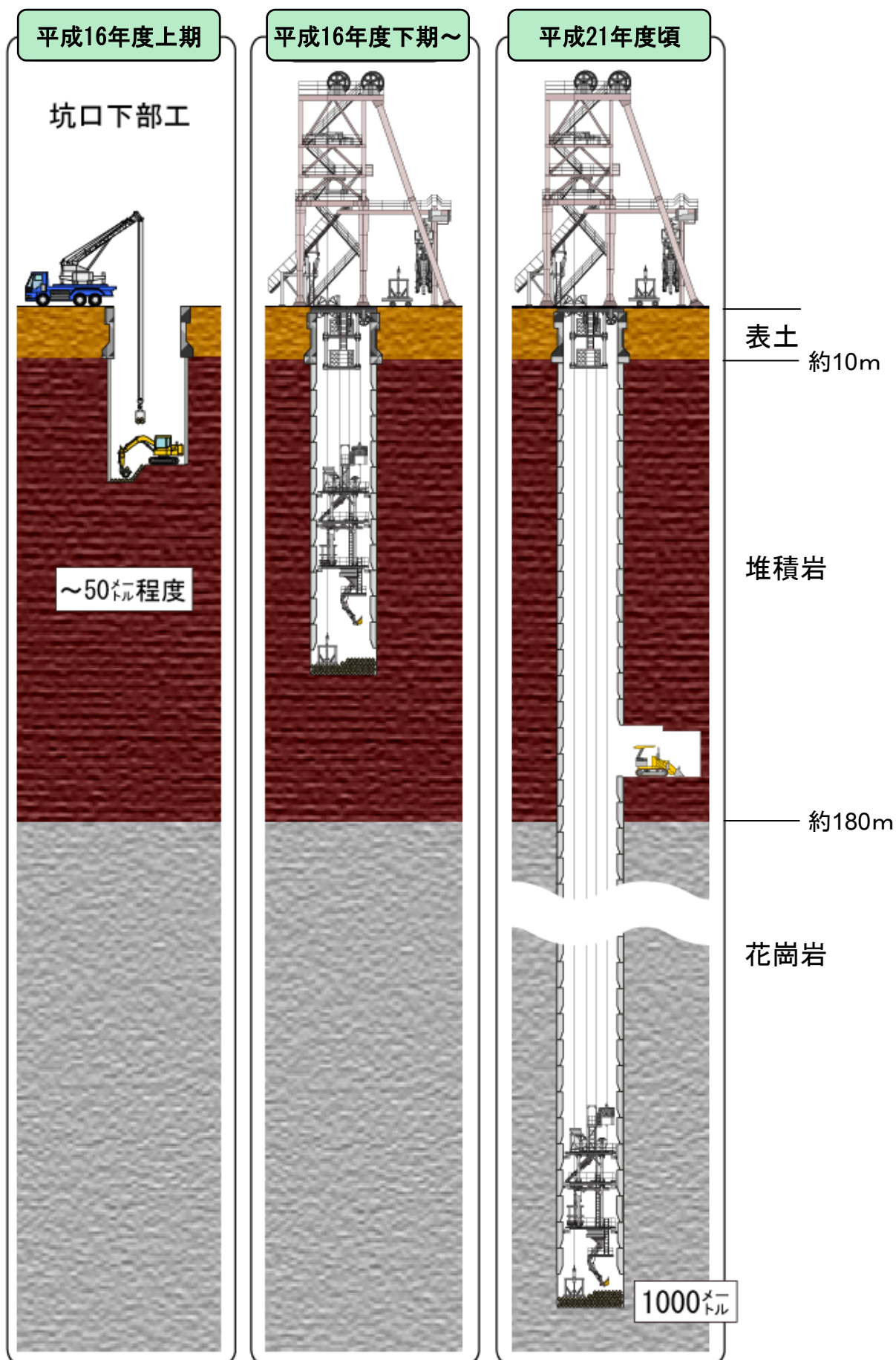
図 4 立坑の掘削工事計画
