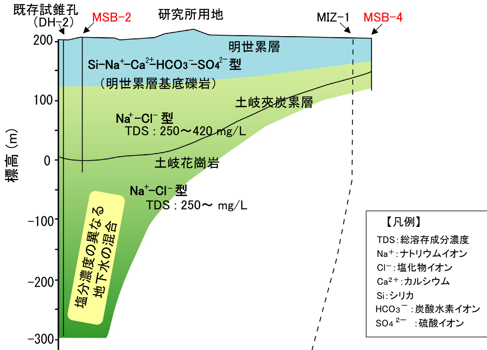
図3 研究所用地の地下の地下水の水質分布
