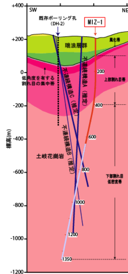
推定した不連続構造分布と深層 ボーリング孔 (MIZ-1) の掘削実績
