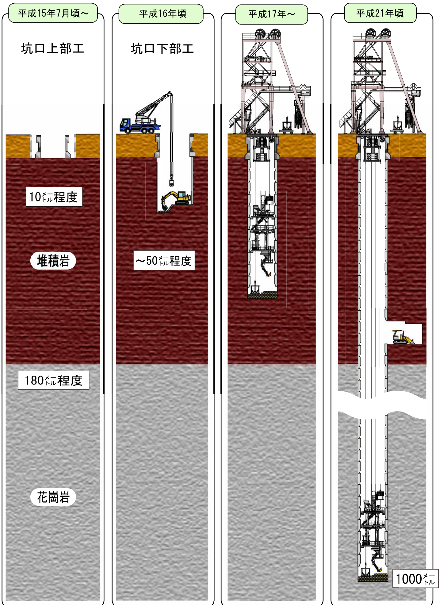
図1 立坑施工概要図
