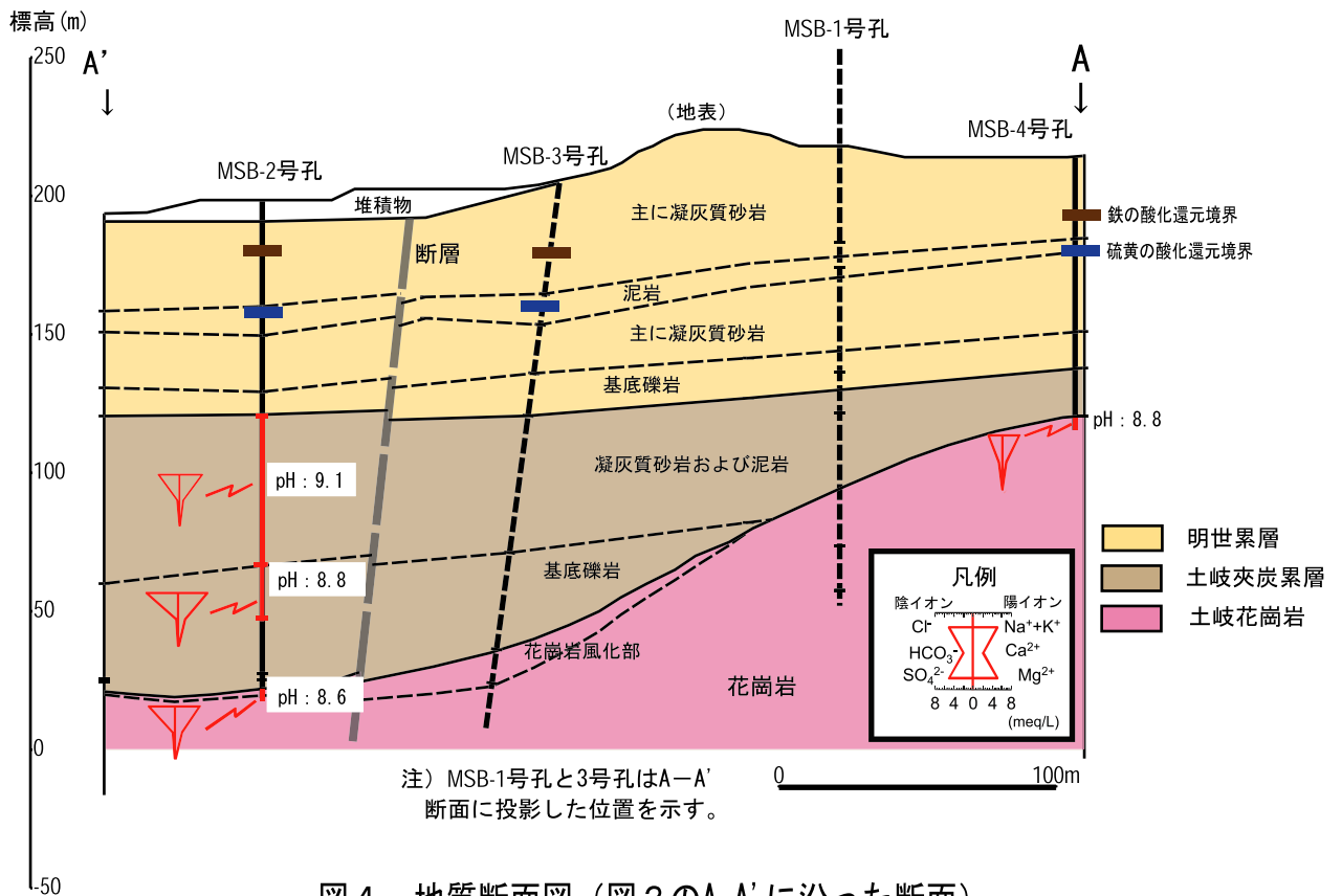
図4 地質断面図 (図3のA-A'に沿った断面)
