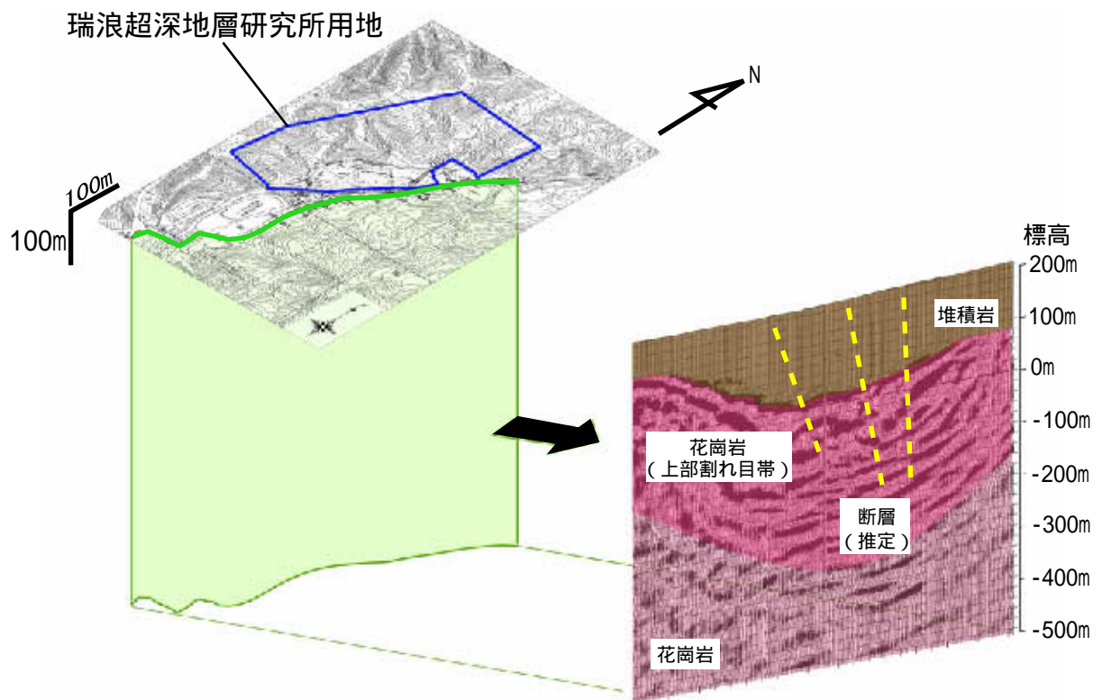
図2 地上物理探査で推定された地質構造
