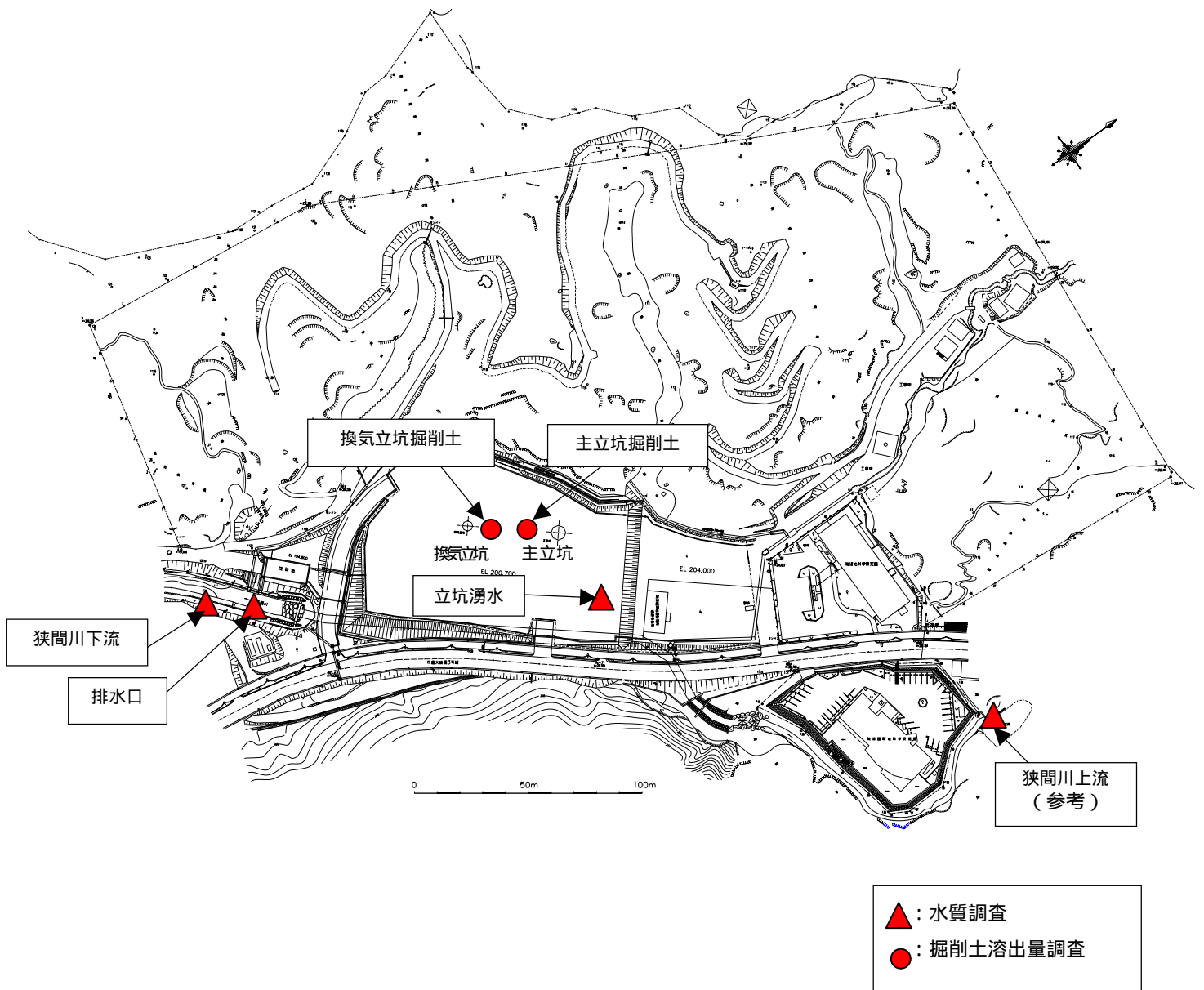
測定位置図
