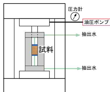
コアからの間隙水抽出装置の概念図
