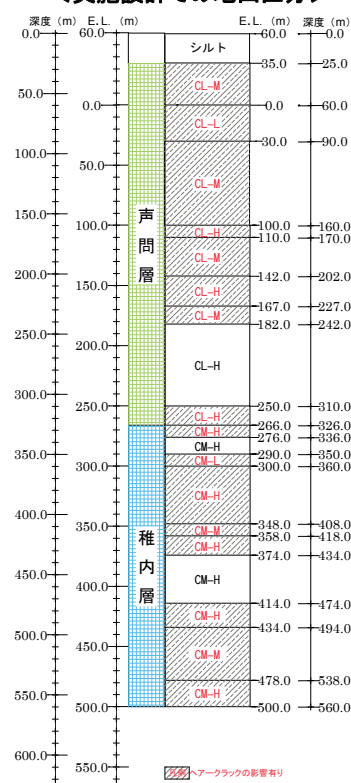
＜実施設計での地山区分＞
