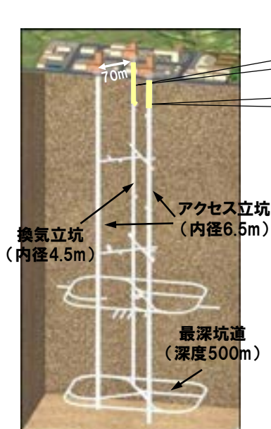
地下施設イメージ (H17.11 立坑掘削開始)
