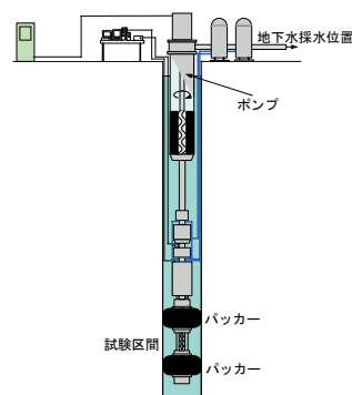
揚水地下水の採水装置の概念図
