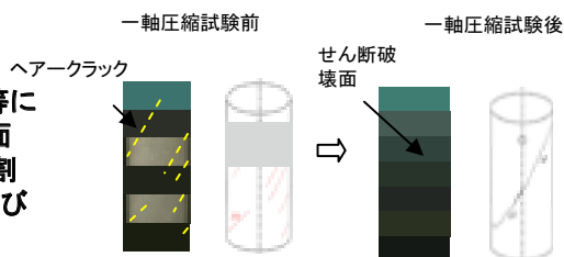
室内試験によるヘアークラックの破断状況
