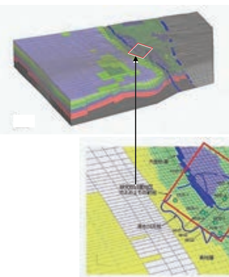
地下水流動解析のため 調査位置図(上)と要素分割(下) 上図の全体の領域は約30km四方
