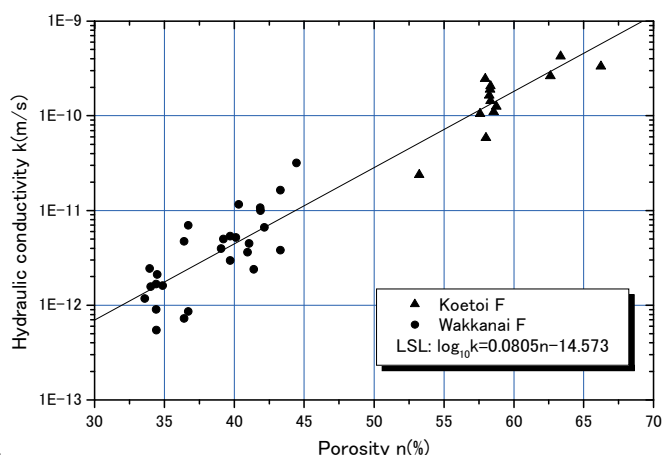
透水係数分布(室内試験)
