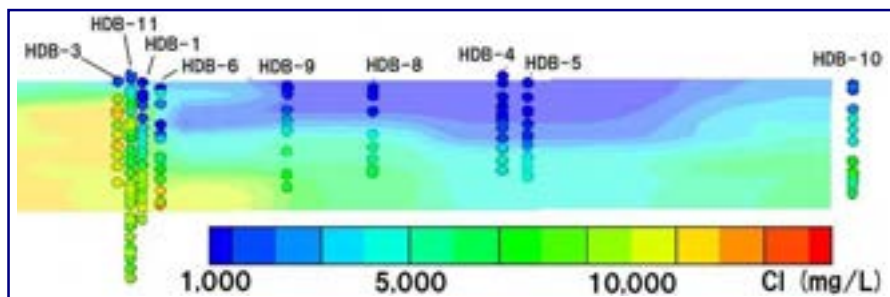
地球化学モデル
