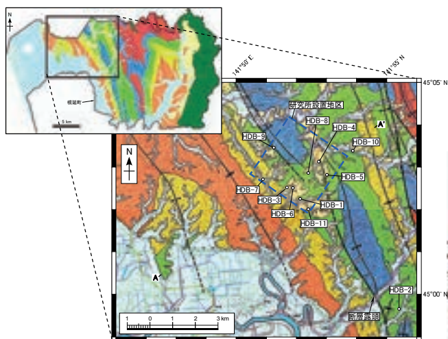
研究所設置地区及び周辺の地質図
