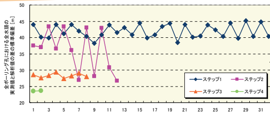
地下水流動特性の不確実性の推移
