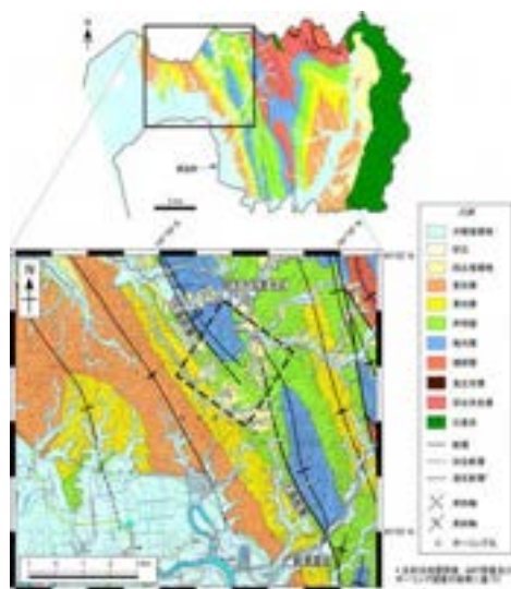
図1 研究所設置地区周辺の地質図
