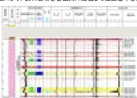
深層ボーリング孔における割れ目の抽出結果の一例
