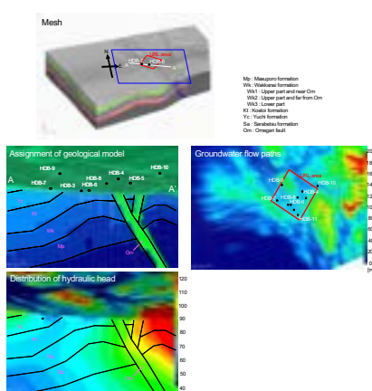
図7 水圧分布と各ボーリング孔(HDB-4, 6, 7, 8, 9, 10, 11)を通る地下水流経路
