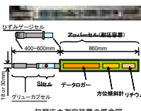
初期応力測定装置の概念図
