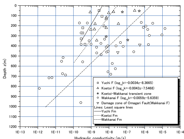
透水係数分布(原位置試験)
