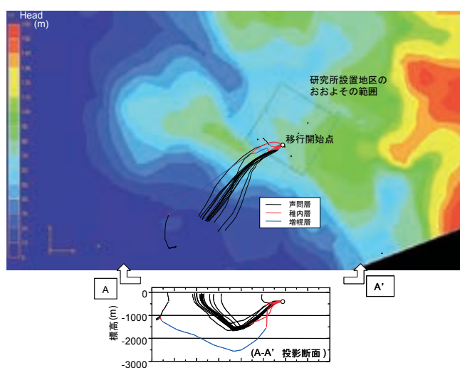
標高-400m断面の全水頭分布と 移行開始点からの地下水流動経路の解析例
