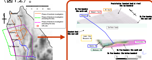
図2 水理地質構造モデルおよび境界条件
