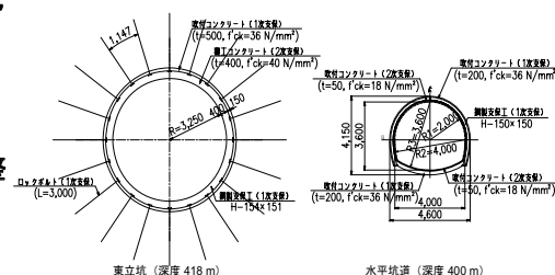
二重支保構造の例
