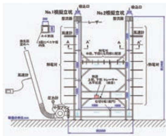
通気挙動模型実験装置の概要
