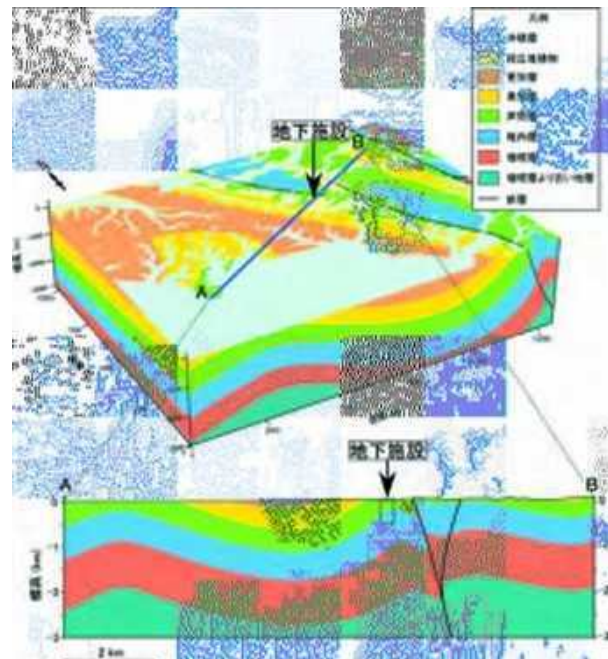
研究所設置地区および その周辺の地質構造モデル
