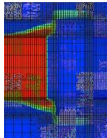
原位置試験閉鎖要素 3次元トレーサ解析結果 (トレーサ濃度分布100日後)
