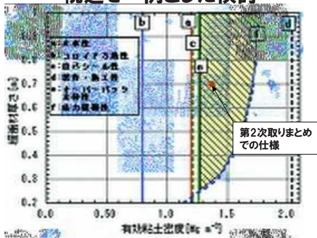
緩衝材設計例(ブロック方式)
