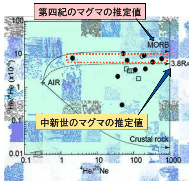
^3\text{He}/^4\text{He} 比と ^4\text{He}/^{20}\text{Ne} 比の関係
