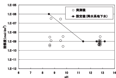
トリウム(Th:アクチノイドIV価)の溶解度の取得結果と降水系地下水での設定結果の比較の一例
