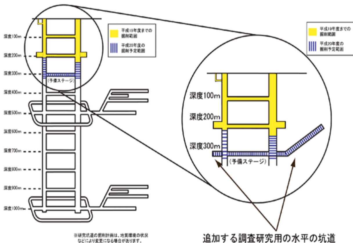
平成20年度の研究坑道掘削範囲図(概念図)
