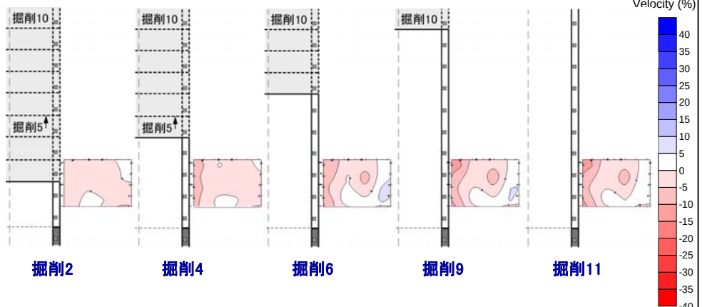
掘削前後の弾性波速度分布の変化率
