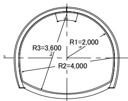
140m調査坑道断面図 支保工厚: 約20cm
