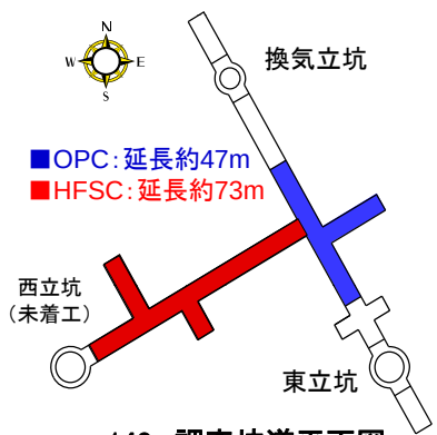
140m調査坑道平面図
