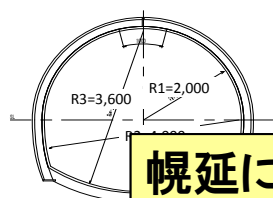
140m調査坑道 支保工厚: 約20cm
