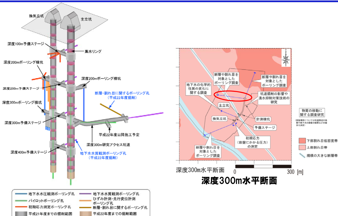
研究坑道におけるボーリング調査などのレイアウト
