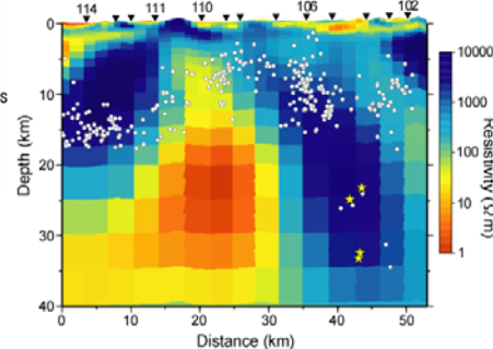
比抵抗構造
