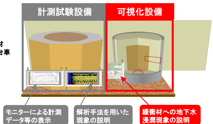
人工バリア長期挙動試験設備の概念図
