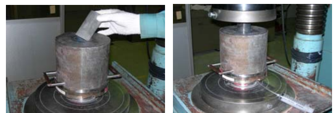
高圧抽出装置によるセメント硬化体からの間隙水の採取状況 (左図:硬化体のセッティング, 右図:載荷及び間隙水の採取)
