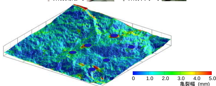
研削により計測した亀裂形状と亀裂幅 (1mm×1mmピッチの計測データ)
