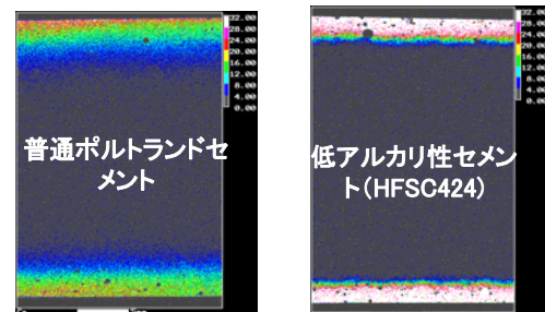
EPMAを用いたセメント硬化体中のセシウムの濃度分布評価例 (図の上下が、溶液との接触面(30日間浸漬)であり、白→ピンク→赤→緑の順で接触面からのセシウムの濃度が低下している)
