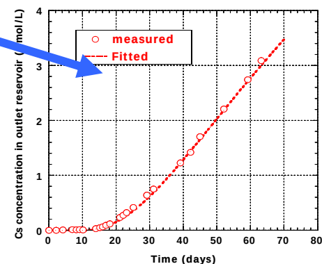
トレーサー破過曲線
