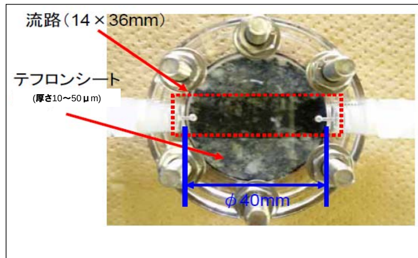
人工平行平板亀裂への高アルカリ性溶液通水試験
