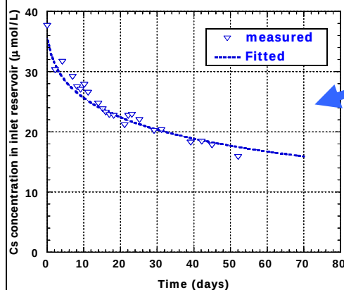
トレーサー減衰曲線
