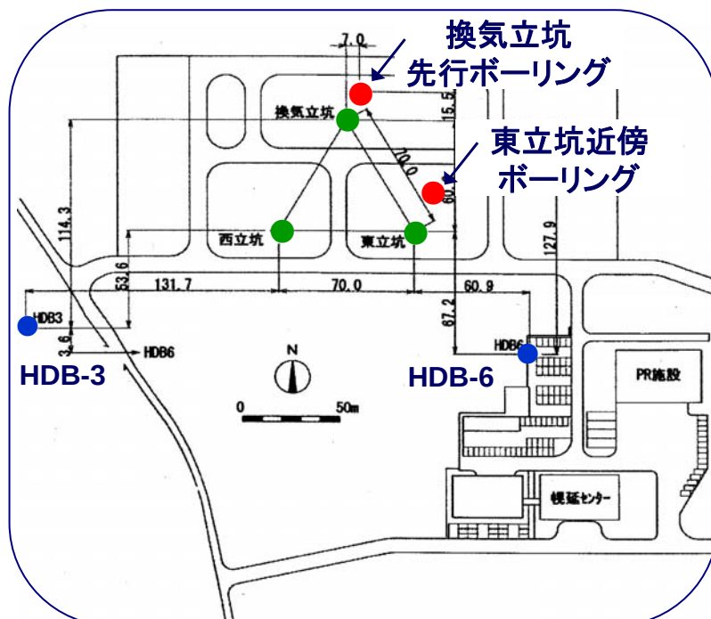
地下施設敷地内でのボーリング調査位置 10
