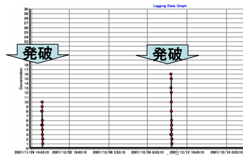
MIU坑道掘削における発破前後の水素濃度の経時変化
