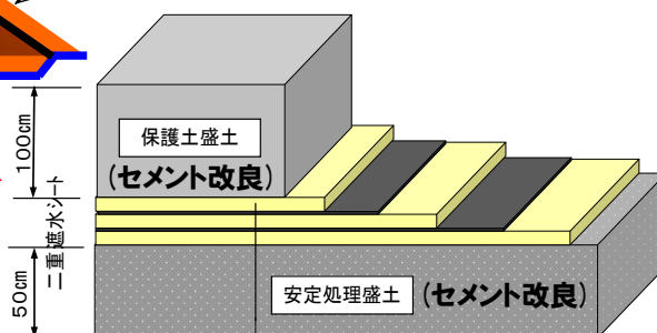
掘削土(ズリ)置場の概念図
