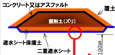
掘削土(ズリ)置場の概念図
