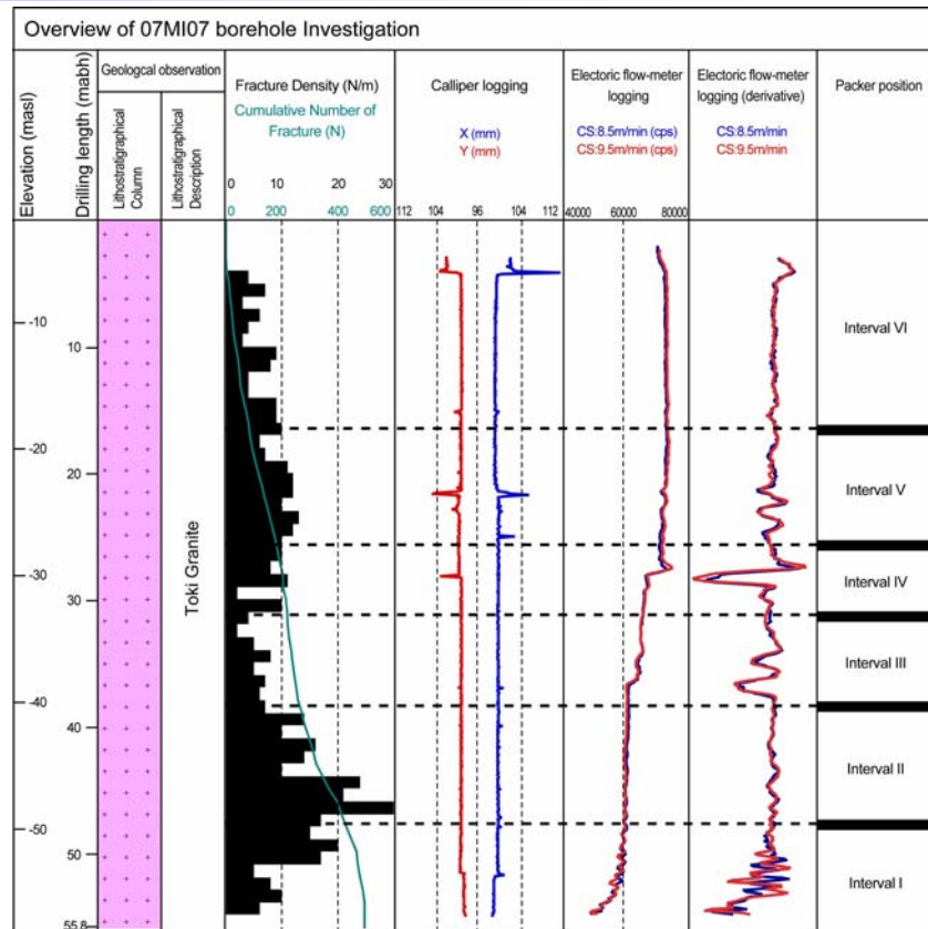
ボーリング柱状図 (07MI07号孔) と測定区間
