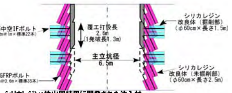
シリカレジン: 地山固結用に開発された注入材。 珪酸ソーダを組成とする溶液の反応によりその効果を発揮する。 地山薬液注入工の概念図
