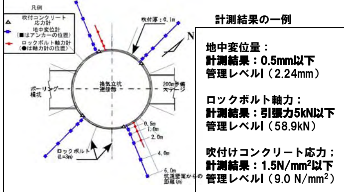
換気立坑接続部における計測配置 *管理レベルはI→IIの順に危険側となる
