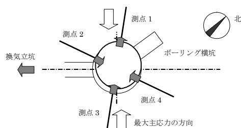
各種計測結果からの推定した主立坑周辺の变形モード
