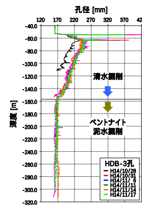
清水掘削とベントナイト泥水掘削との比較
