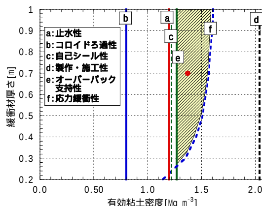
ブロック方式を一例とした 緩衝材の試設計例
