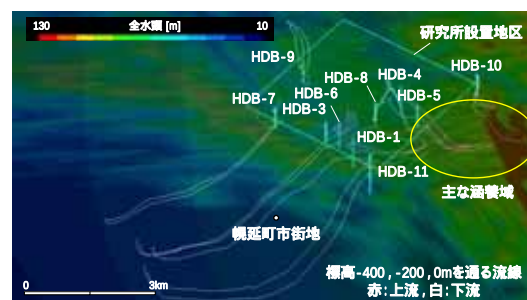
地下水流動解析結果の一例
