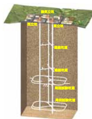
地下施設の基本レイアウト
