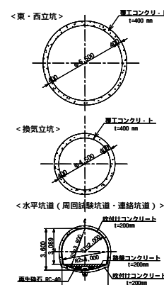
地下施設の基本レイアウト
