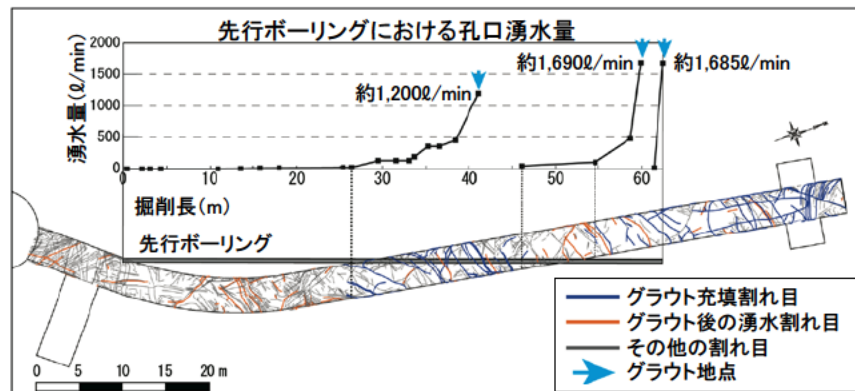
先行ボーリング調査における湧水量と壁面地質
