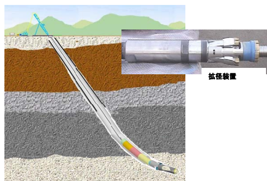
コントロールボーリングの概念
