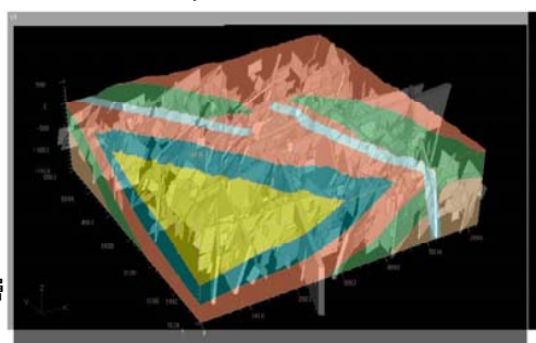
3次元地質構造モデル (研究所設置地区)
