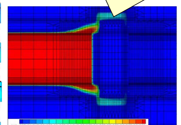
粘土プラグ内のトレーサー濃度分布の解析結果
