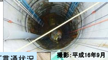
主立坑掘削状況
