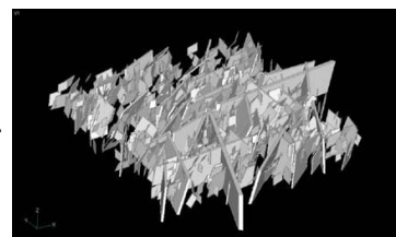
割れ目帯ネットワーク
