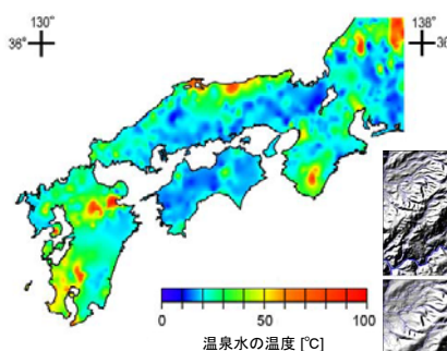
西南日本の泉温コンター図
