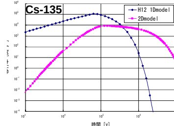
掘削影響領域からの移行率の経時変化
