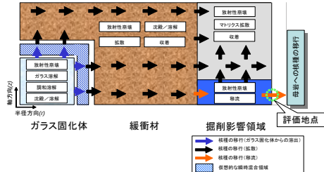
2次元人工バリア中核種移行モデルの概念図
