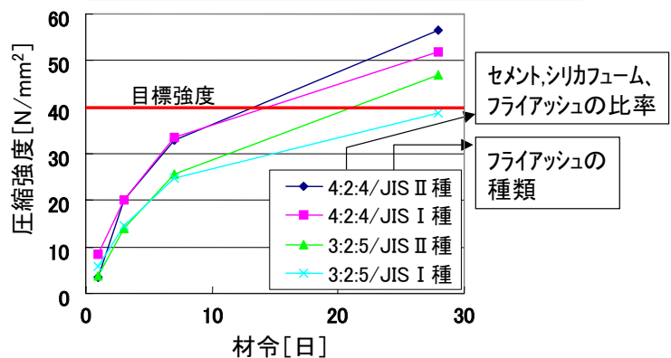
低アルカリ性コンクリートの圧縮強度
