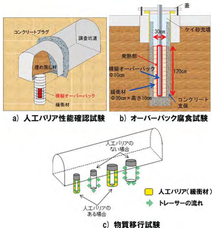
図 3.2-1 実際の地質環境における人工バリアの適用性試験
