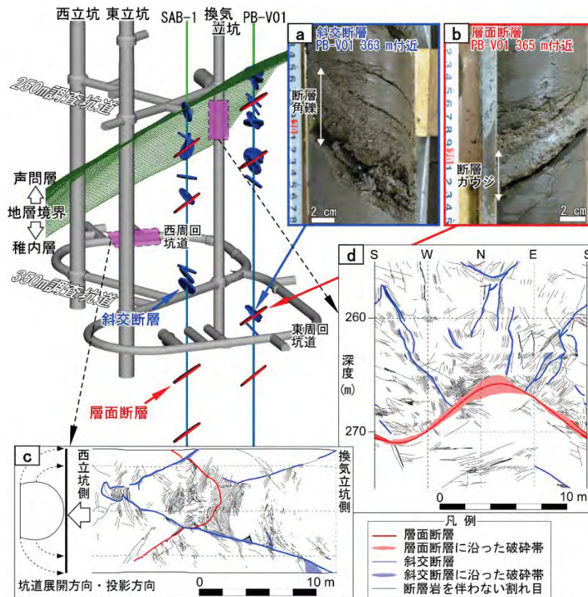
図 1.1-1 幌延深地層研究センターの地下施設のレイアウトと先行ボーリングで確認された断層および断層の交差関係が観察された坑道壁面の展開図（原子力機構, 2017） 19)
