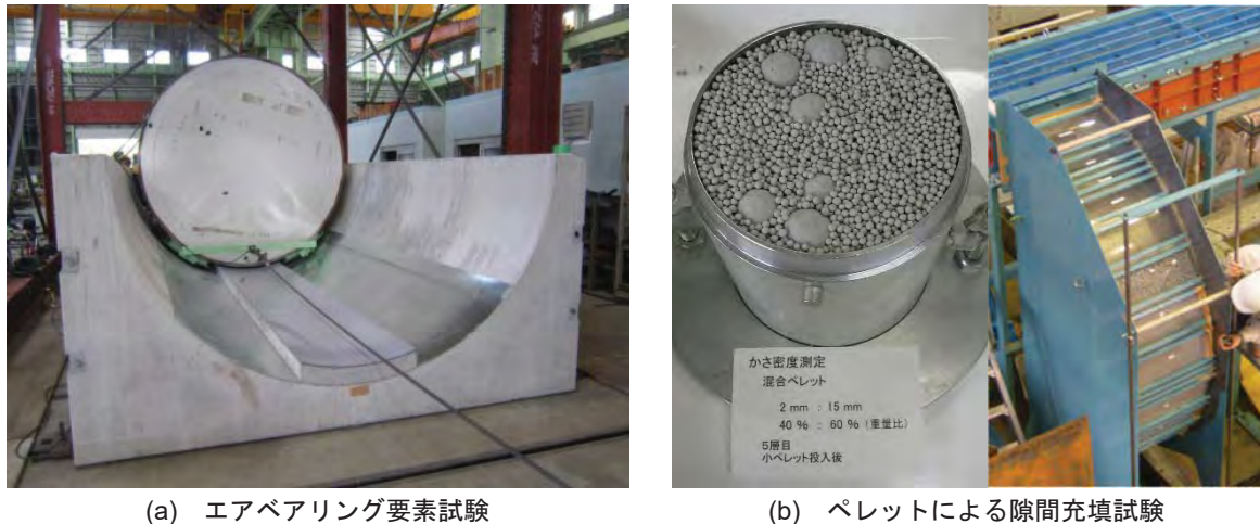
図 4.2.2.1-4 PEM の搬送・定置技術、隙間充填技術の整備状況
