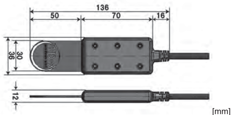
図 4.1.2.2-24 含水率センサー寸法
