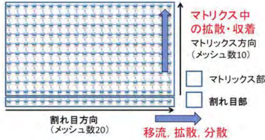
図 4.1.3.2-2 解析モデル概念図：(a)均質系、(b)不均質系 (原子力機構、2016) 24)
