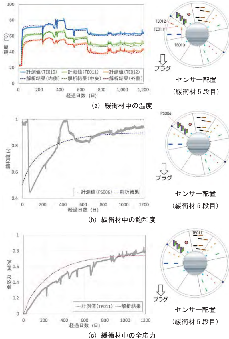
図 4.1.1.5-20 THM 連成解析結果と緩衝材中の計測値との比較
