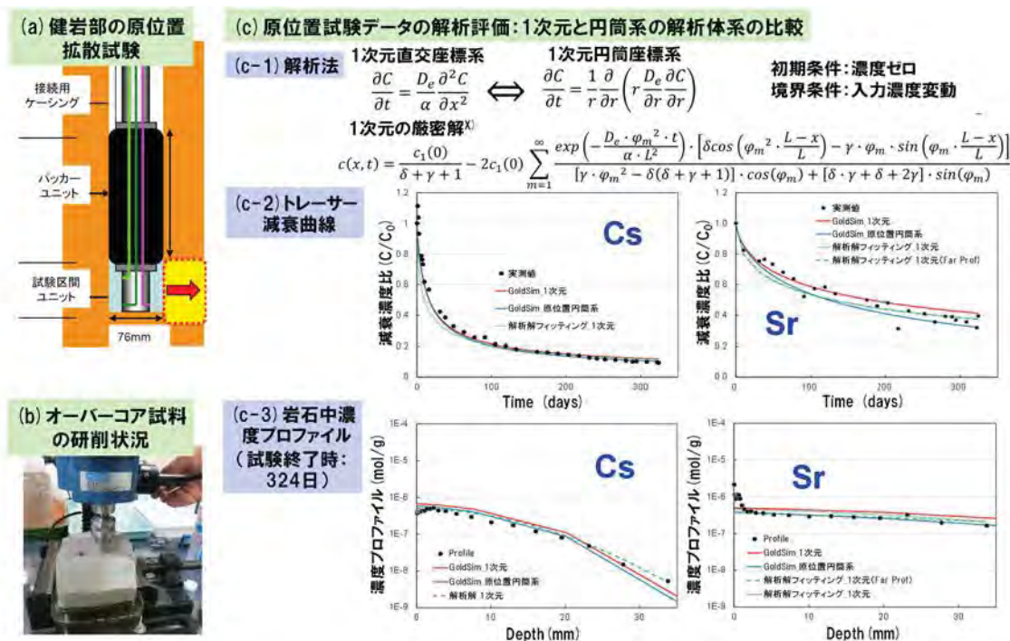
図 4.1.3.1-2 D-05 孔の原位置拡散試験の試験体系(a)、オーバーコア試料の分析状況(b)、および 1 次元直交座標系と 1 次元円筒座標系での解析結果の比較(c)
