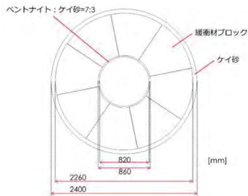
図 4.1.1.3-2 緩衝材ブロック断面
