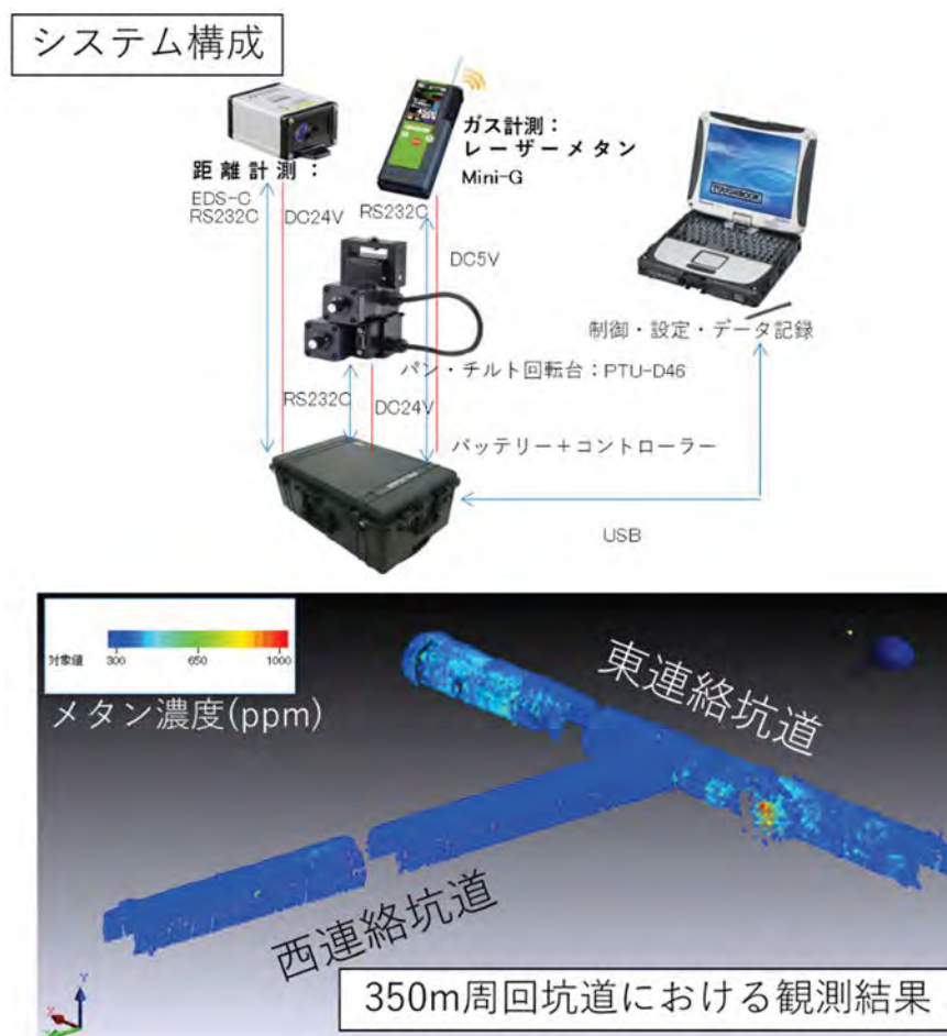
図 1.3-6 新しく開発した計測装置のシステム構成（上）と計測例（下）
