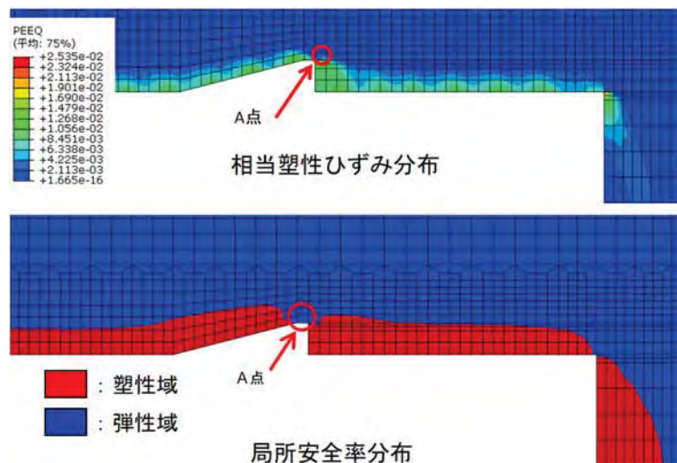
図 4.1.1.2-11 掘削解析結果（プラグ切り欠き部）
