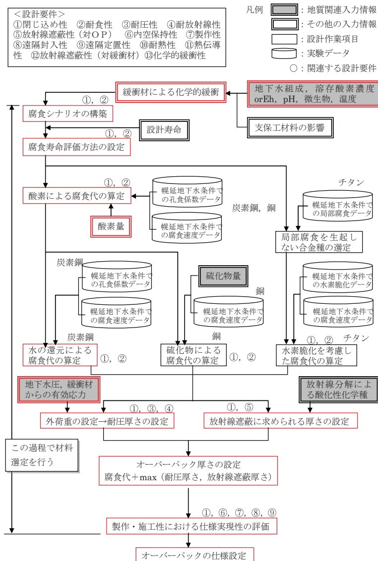
図 4.1.1.1-3 オーバーバック設計フロー
