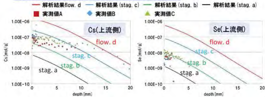
図 4.1.3.2-3 定流量通水試験結果の解析例 (原子力機構、2016 24) を一部加工)
