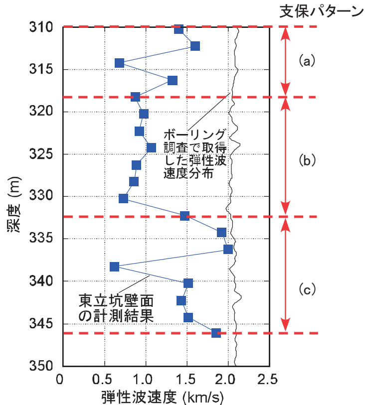
図 4.2.1.2-5 東立坑深度 310 m～346 m における弾性波速度の分布 (支保パターンの(a)～(c)はそれぞれ図 4.2.1.2-4 (a)～(c)に対応している)
