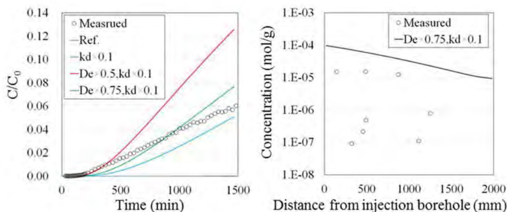
図 4.1.3.2-12 Cs の解析結果 (a)定常入力条件、(b)割れ目表面における Cs 濃度 29)
