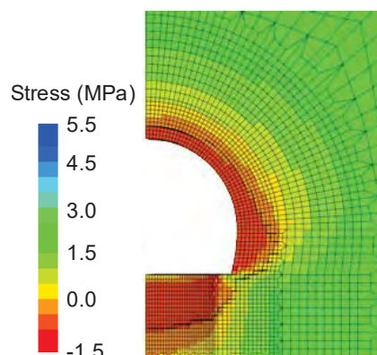
図 2-9 最小有効主応力の分布（圧縮応力が正）
