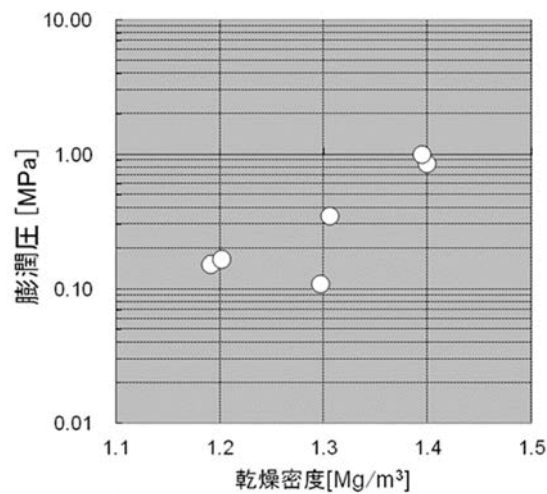
図 4.1.1.2-4 乾燥密度と膨潤圧の関係
