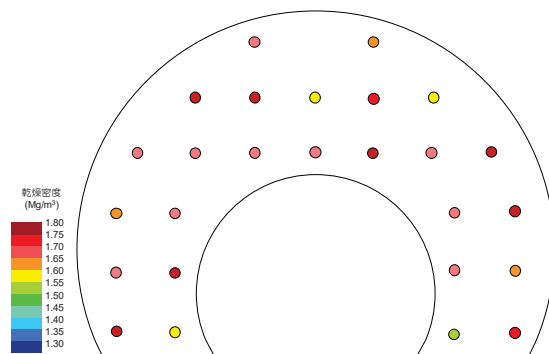
図 4.2.2.1-13 吹付け面からのサンプリング位置と乾燥密度分布の一例
