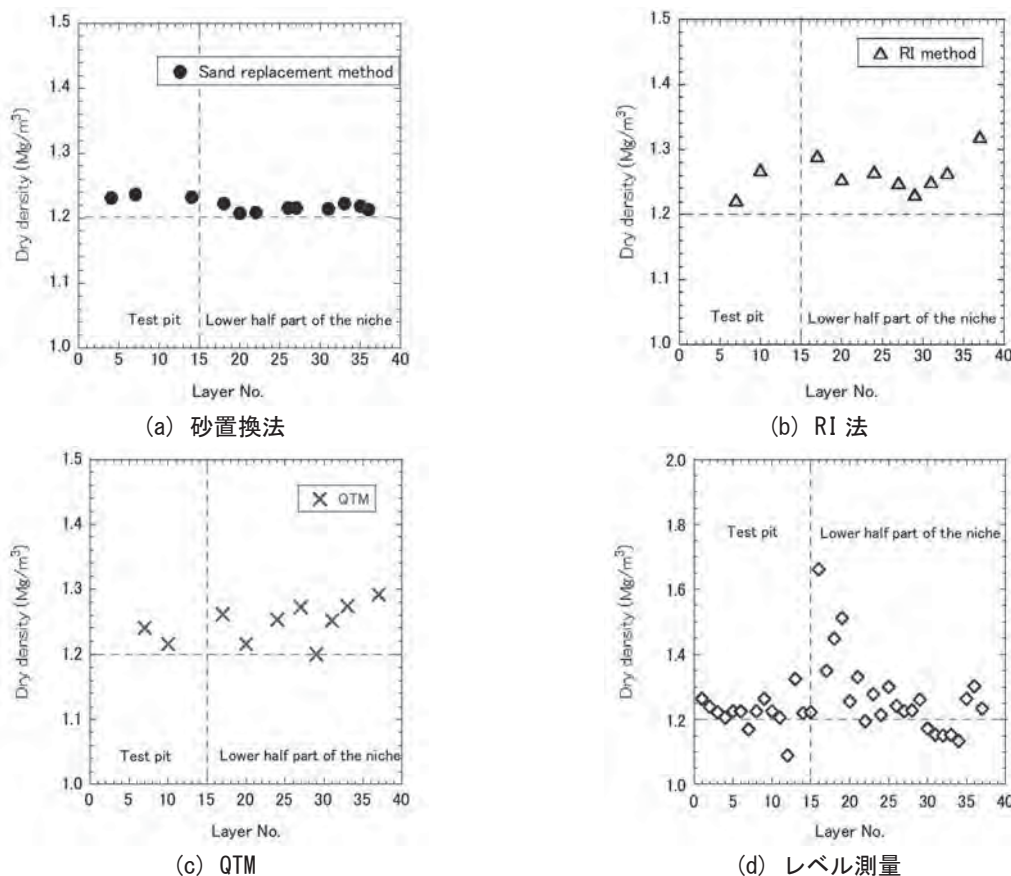
図 4.1.1.4-6 各手法による乾燥密度の測定結果
