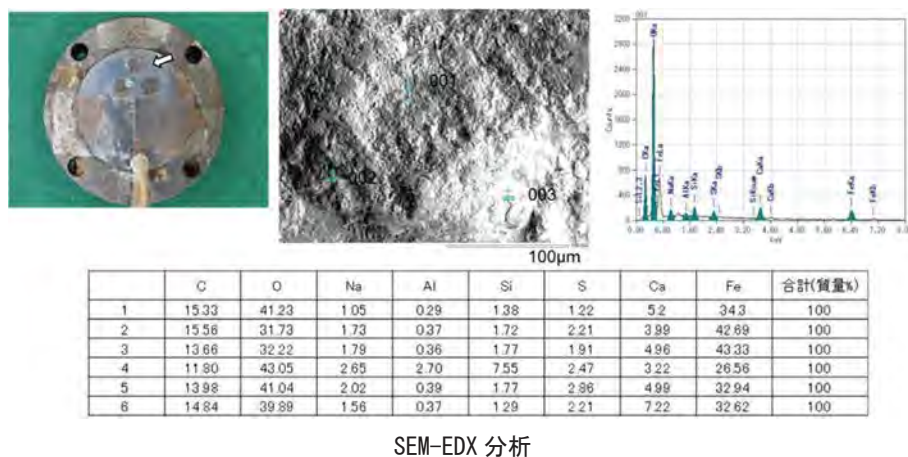
図 4.1.2.2-10 回収後の三電極式センサーの腐食生成物分析
