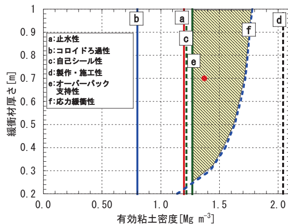
図 4.1.1.1-2 ブロック定置方式による緩衝材単独の仕様範囲
