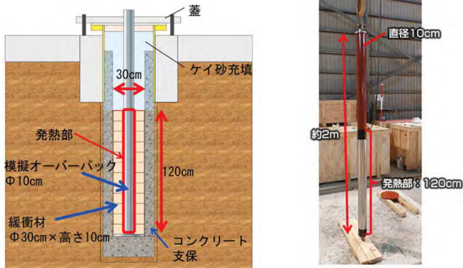
図 4.1.2.1-1 オーバーパック腐食試験の模式図（左）と模擬オーバーパックの外観（右）
