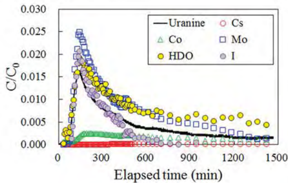
図 4.1.3.2-10 割れ目帯を対象としたトレーサー試験結果
