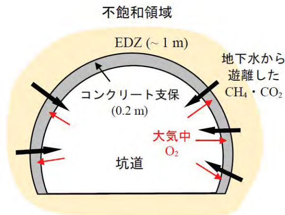
図 2-14 EDZ の化学環境に関する概念モデル
