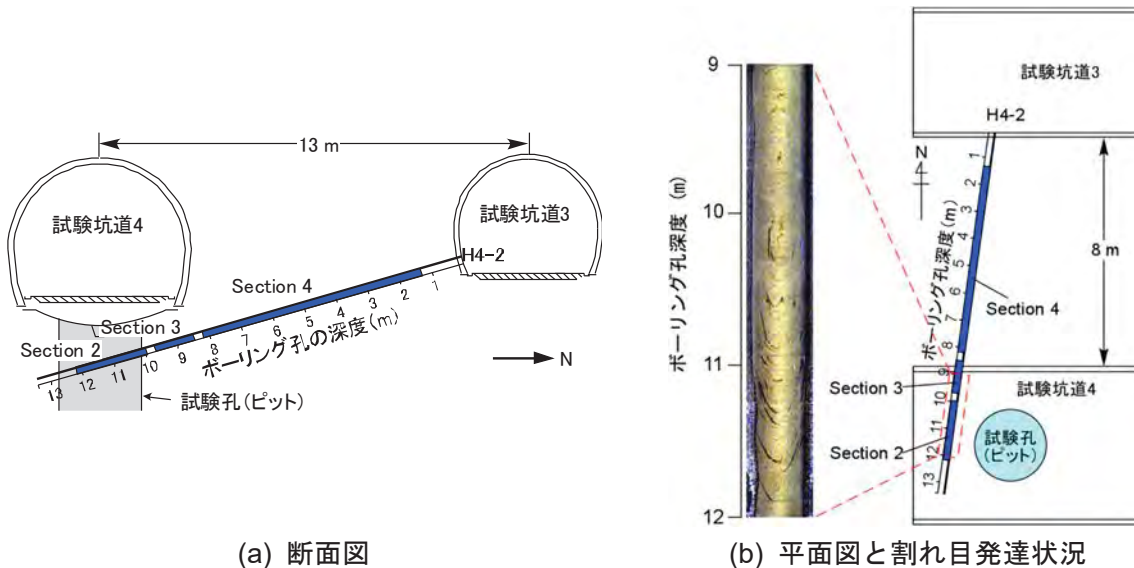
図 2-15 透水試験レイアウトとピット周辺の割れ目発達状況
