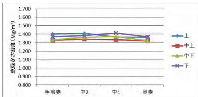
図 4.2.2.1-15 地上でのペレット充填試験後の乾燥密度の分布例 15)
