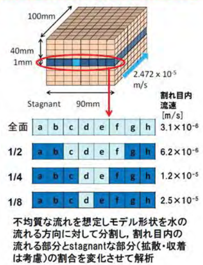
図 4.1.3.2-2 解析モデル概念図：(a)均質系、(b)不均質系 (原子力機構、2016) 24)
