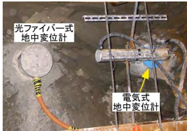
図 4.2.1.2-10 地中変位計設置状況写真
