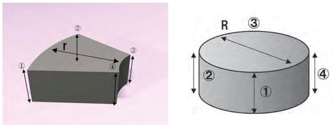
(a) 扇型ブロック
