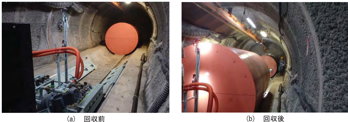
図 4.2.2.1-29 試験坑道 2 における模擬 PEM の回収試験の様子
