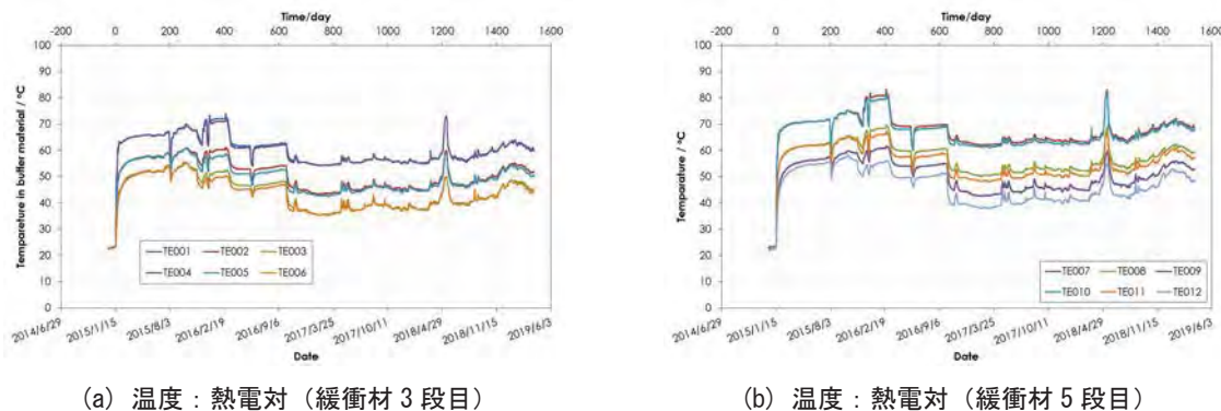
図 4.1.1.5-3 温度計測データ（熱電対）
