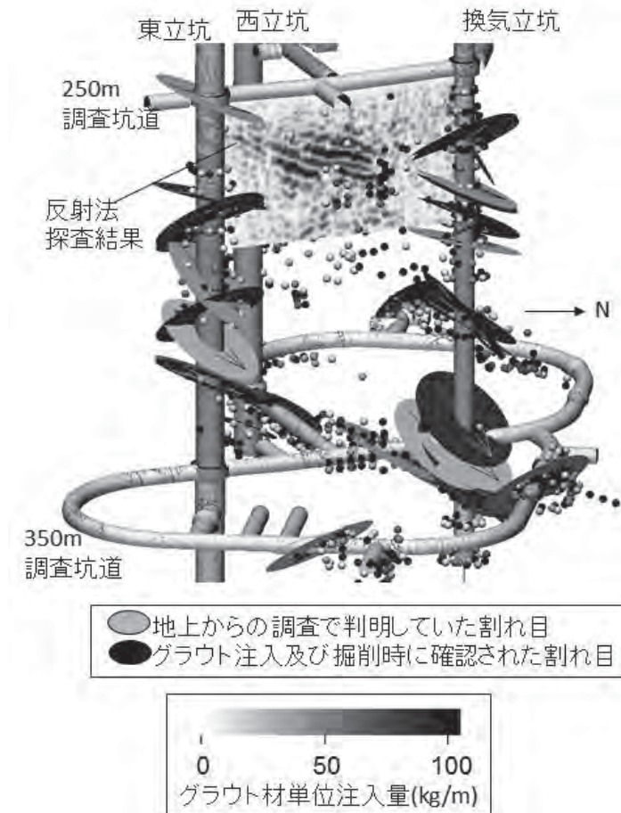
図 4.2.1.2-3 構築した可視化システムによる坑道周辺の断層分布の更新状況
