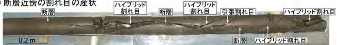
図 1.1-5 コアに認められる断層近傍の割れ目のタイプと DI の関係 (Ishii, 2016) 16)
