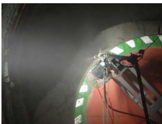
図 4.2.2.1-25 上部開放部の模擬 PEM 近傍の充填材に対するトルネードノズルの効果
