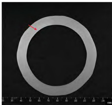
図 4.1.1.3-8 マクロ組織試験結果
