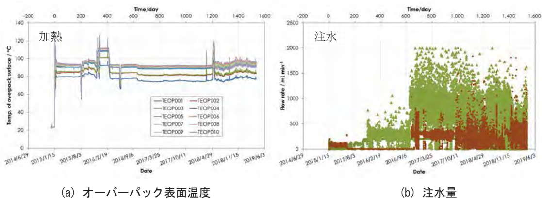
図 4.1.1.5-2 加熱・注水データ
