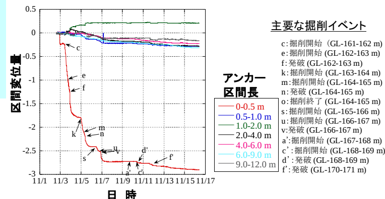
光ファイバー式変位計の区間変位の経時変化
