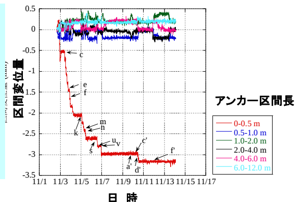
電気式変位計の区間変位の経時変化
