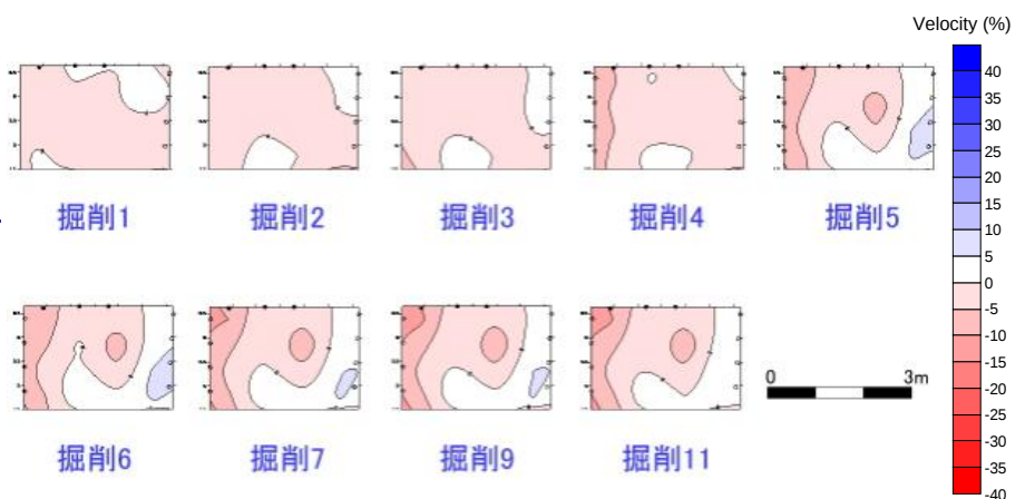
掘削前後での弾性波速度の変化率の分布
