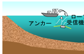
海域電磁探査調査模式図
