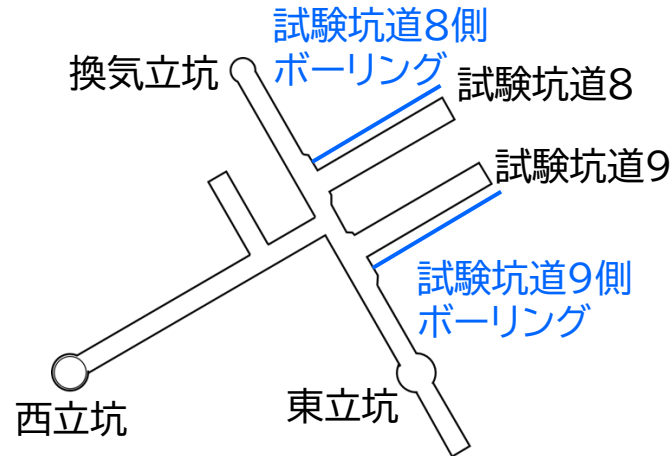
500m調査坑道レイアウト
