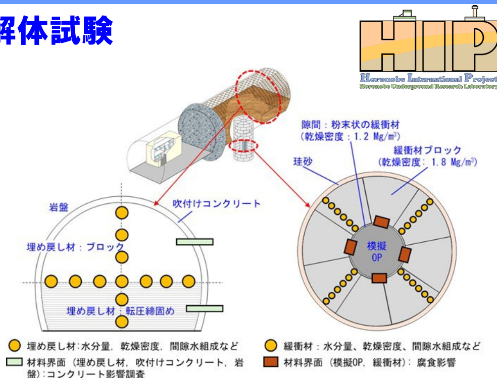
人工バリア性能確認試験の解体試験計画の概要 (大野, 2024)
