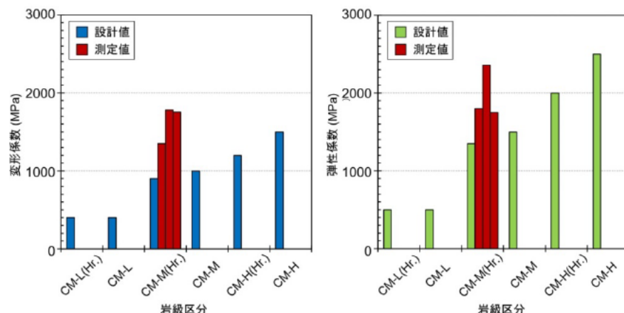
図1 平板載荷試験の結果(350m調査坑道)
