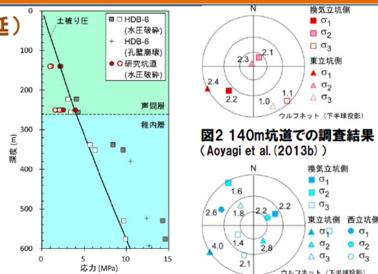
図1 地上からの調査結果と坑道内での調査結果の比較 (after Aoyagi et al. (2013b))
