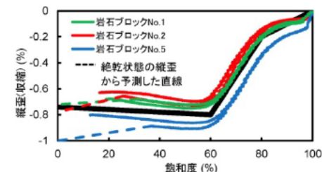
図2 乾燥収縮試験結果 (原子力機構(2013))
