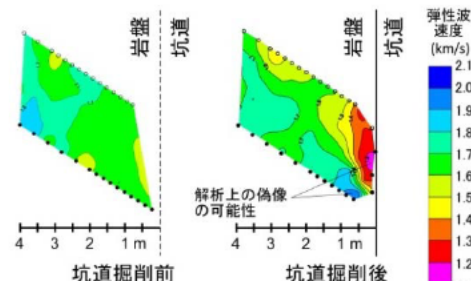
図2 弾性波トモグラフィ結果 (Aoyagi et al. (2013a))
