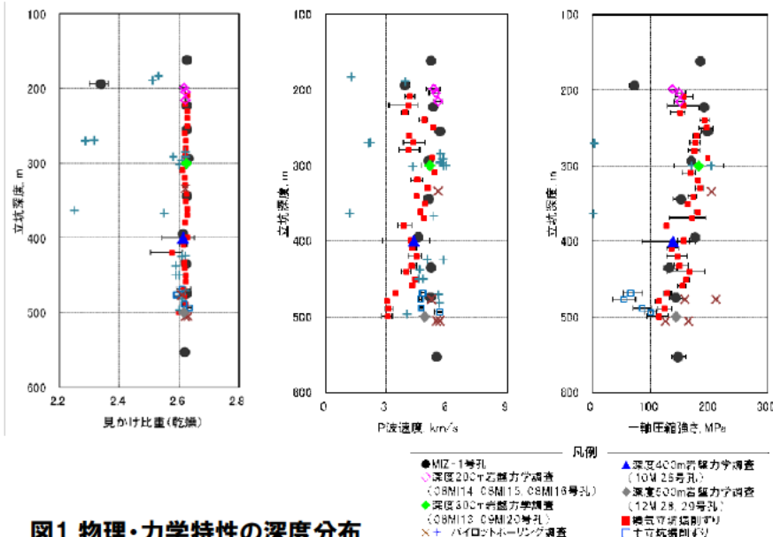
図1 物理・力学特性の深度分布
