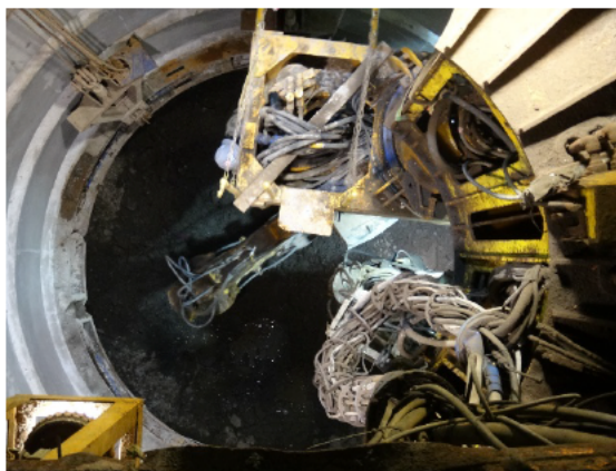
掘削状況 (換気立坑) (平成26年2月12日撮影)
