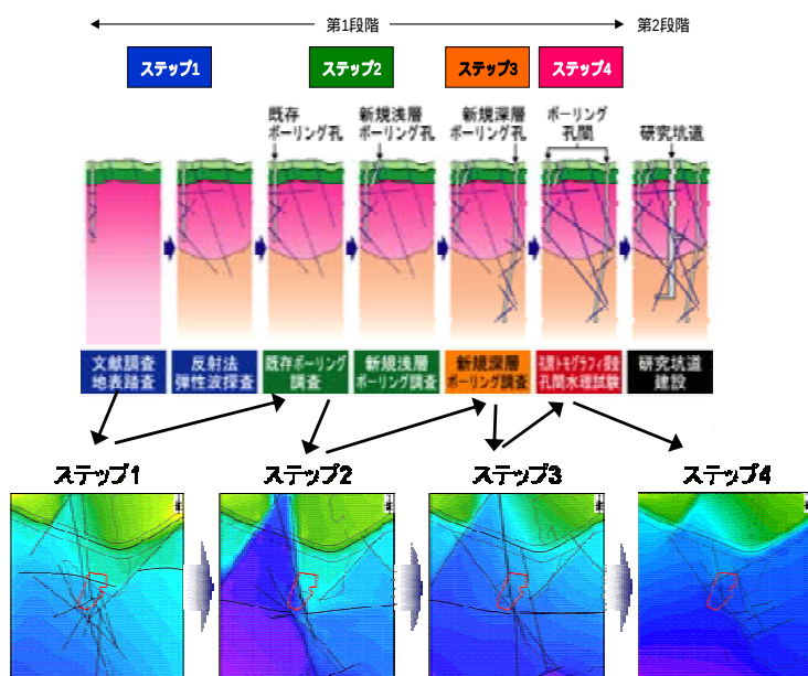
地下水流動解析結果(感度解析結果の一例)
