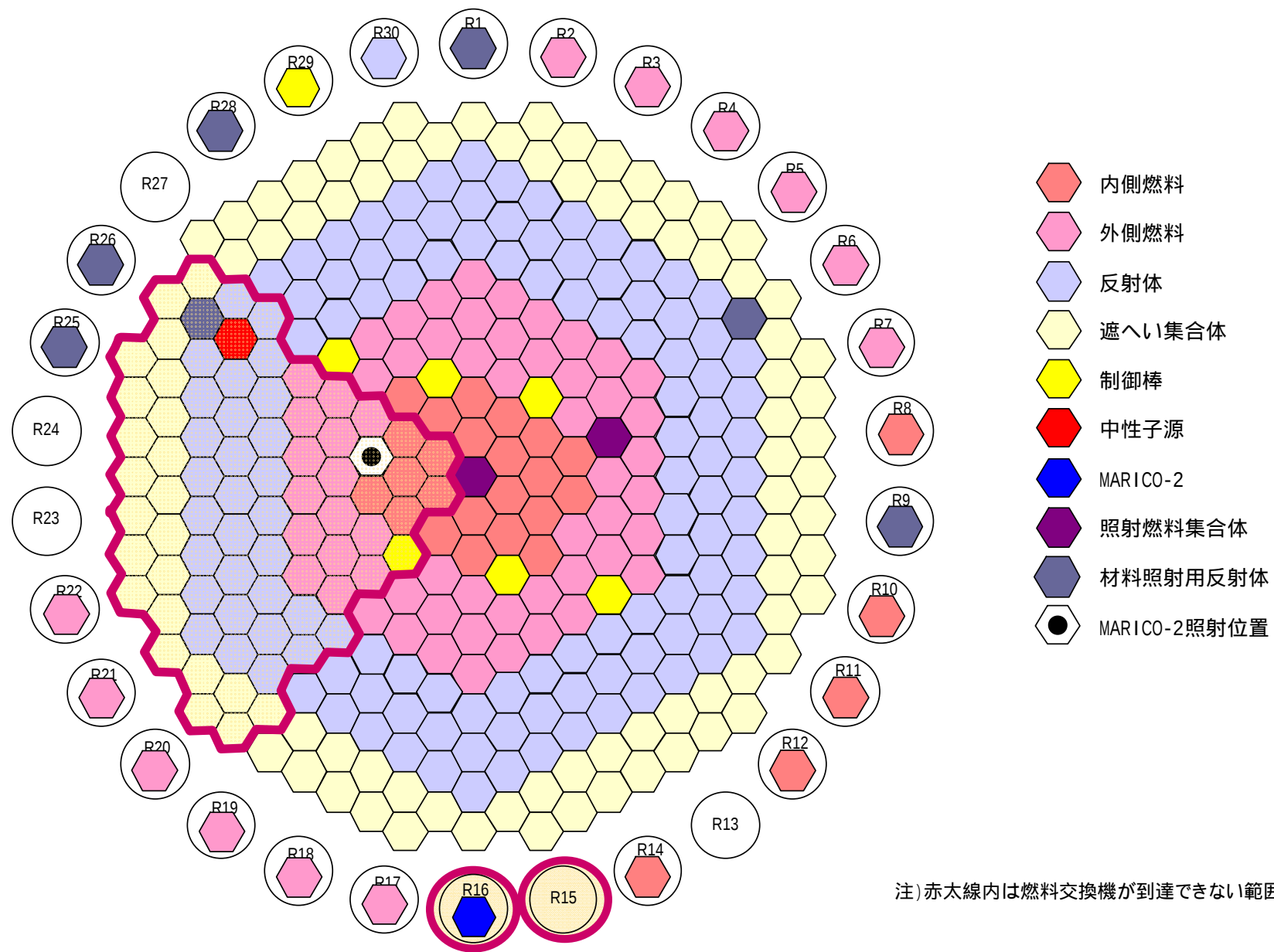
別添図4 炉心構成と燃料交換機が到達できない範囲
