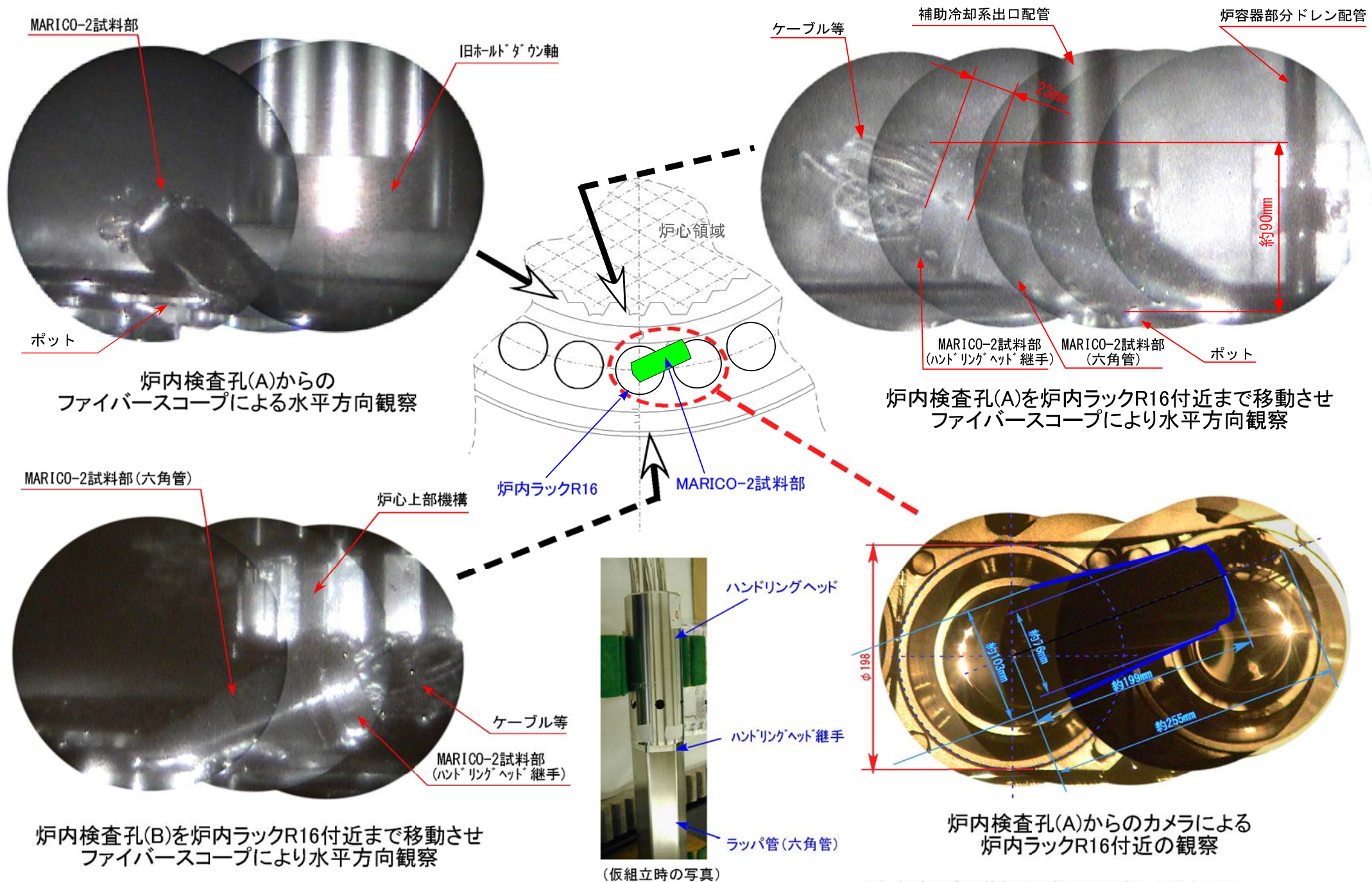
別添図3 炉内ラックR16上部のMARICO-2試料部観察写真
