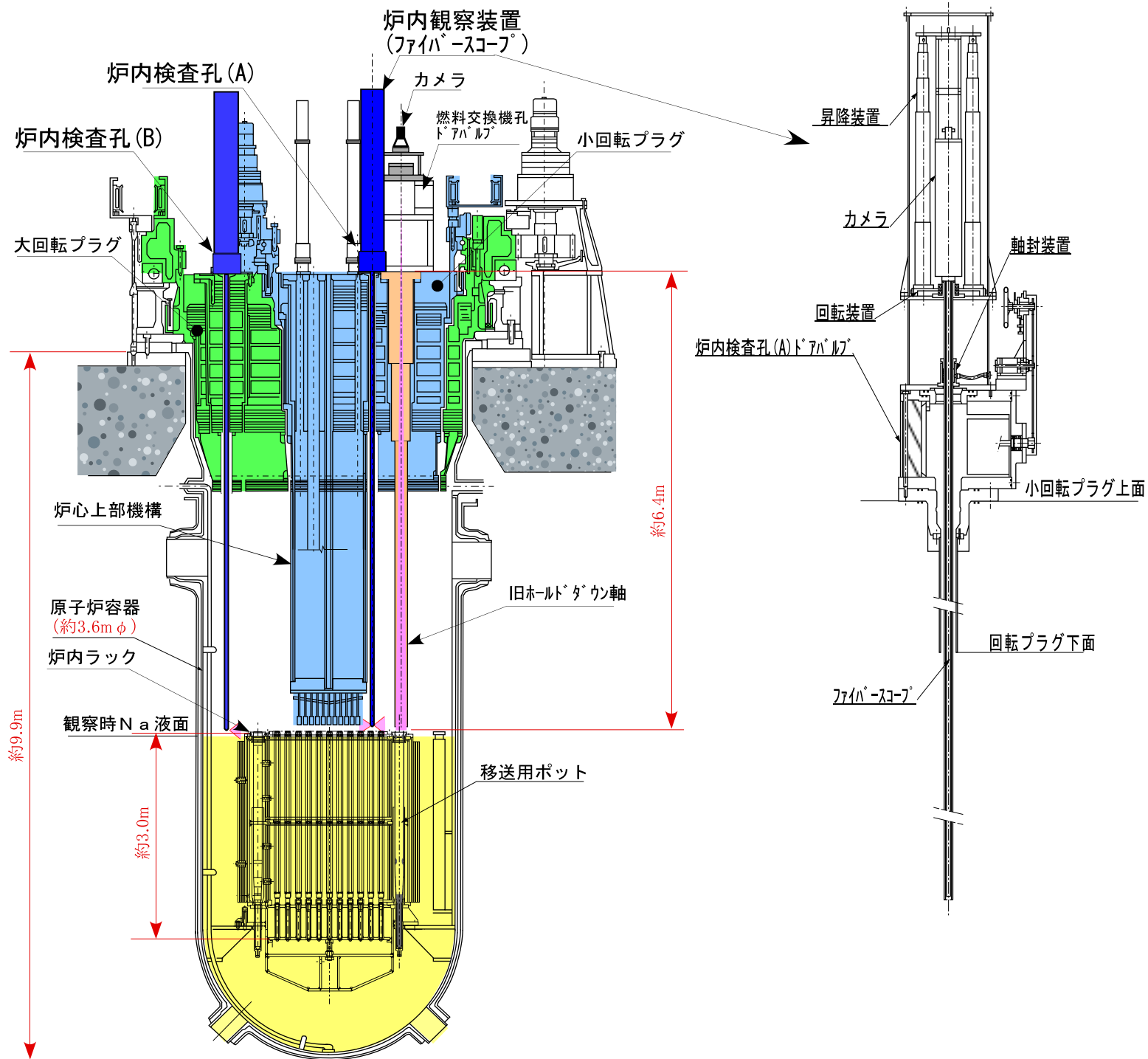
別添図2 原子炉容器内の観察概要図
