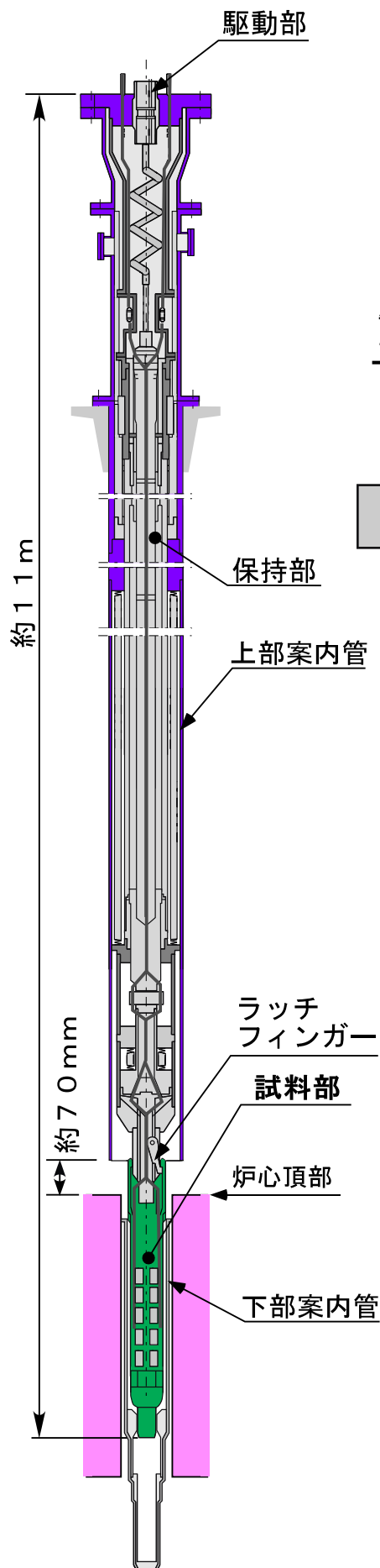
照射時の保持部と試料部の接続状態
